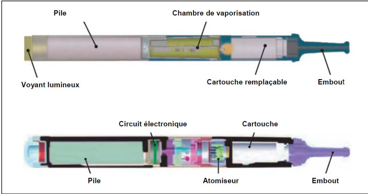
Figure 1 La cigarette électronique et ses composants
